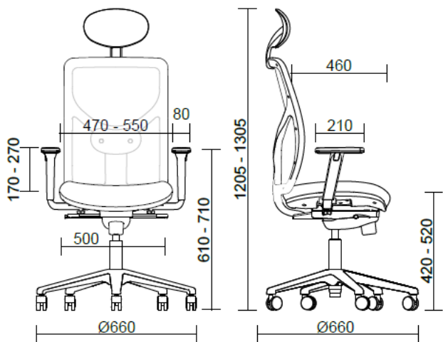
SIÈGE OPÉRATIONNEL AVEC TÊTIÈRE ET ACCOUDOIRS 2D
